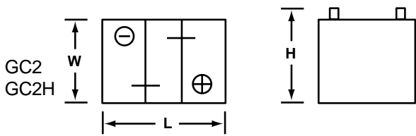
FIG. 2 (6-VOLT 3 CELL)
