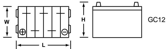
FIG. 32 (12-VOLT 6 CELL)
